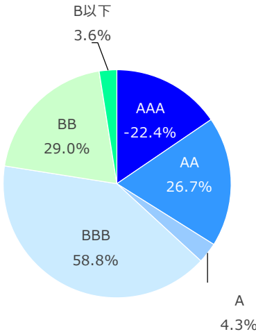
格付分布
