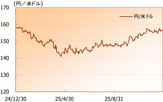
為替の推移
